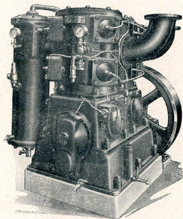
Compresor de aire Atlas - Tipo OKS
